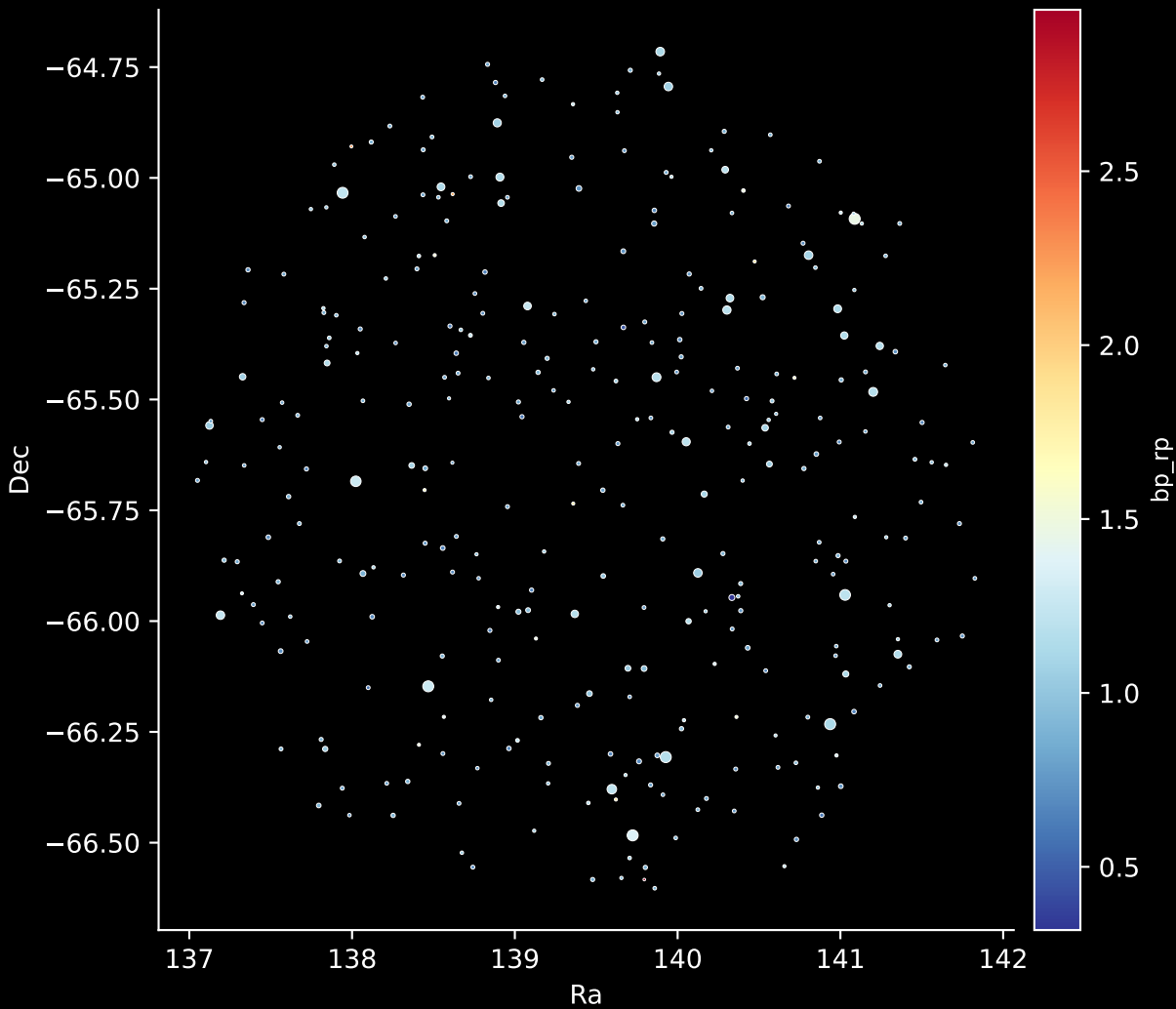
GALAH DR4 Field: [7042] Stars: 311
