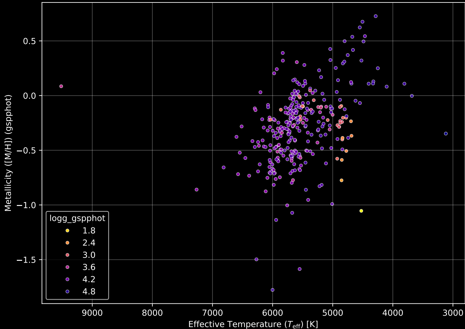
GALAH DR4 Field: [7042] Stellar Population Parameters (n= 311)
